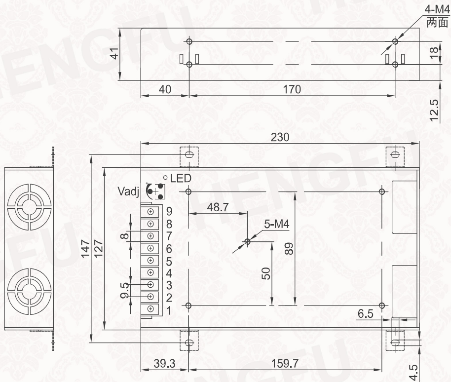
机壳 Frame
